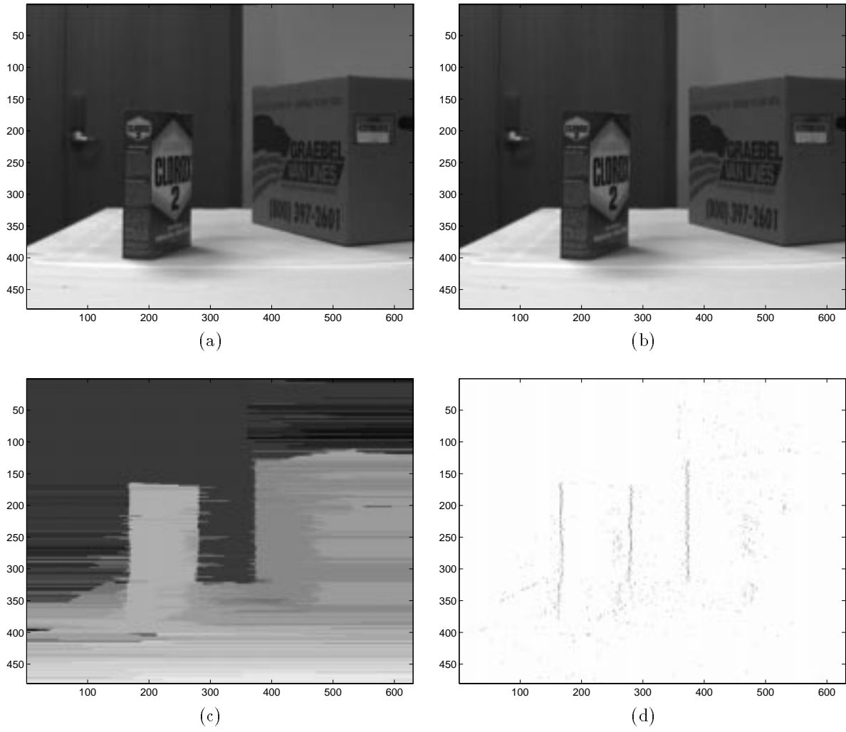
Figure 5.7: (a) Right image. (b) Left image. (c) Disparity map. (d) Depth discontinuities.
